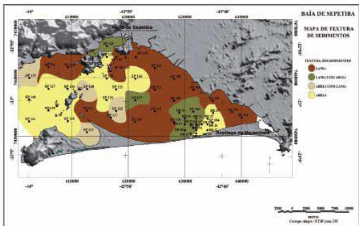
Mapa 3 - TEXTURA DOS SEDIMENTOS MARINHOS NA BAÍA DE SEPETIBA Fonte: Pinto et al. (2018)
